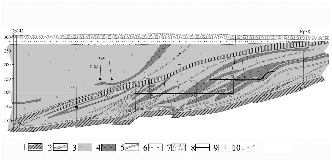
Рис. 1. Геологічні розрізи родовищ калійних солей Передкарпатського прогину (виконав Ю.Ю. Садовий за матеріалами С.С. Корія)
