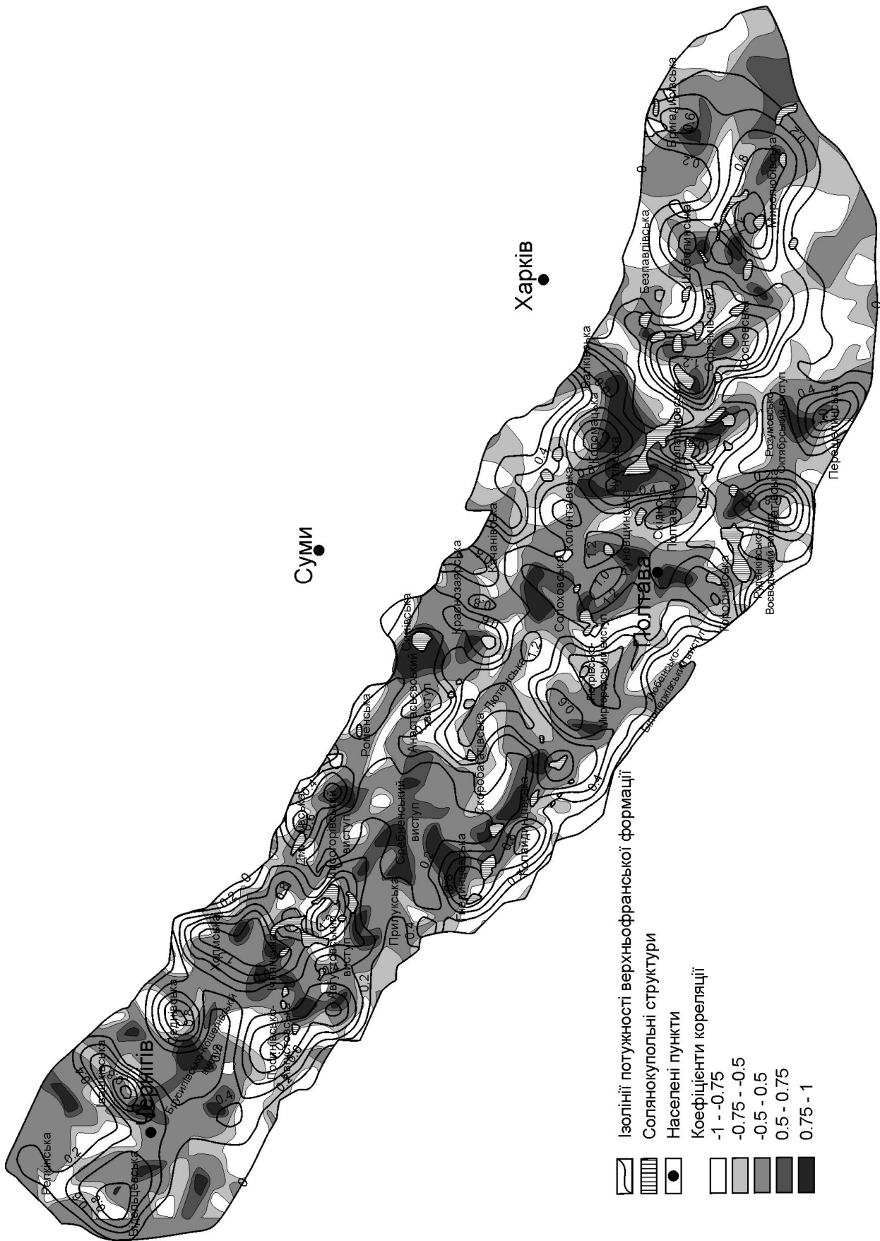
Рис. 3. Кореляція потужності верхньофранківської соленосної формації та поверхні підстилаючих підсоленосних утворень
