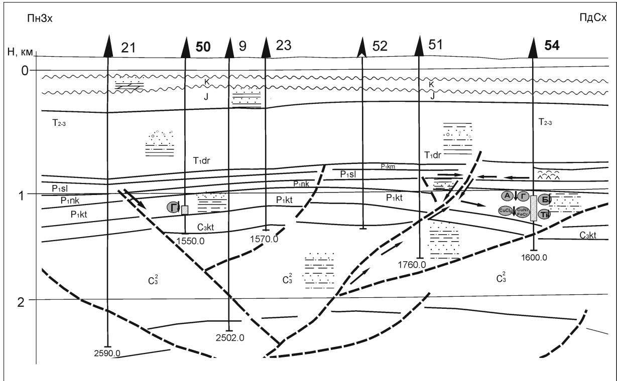
Рис. 5. Сейсмогеологічний розріз
